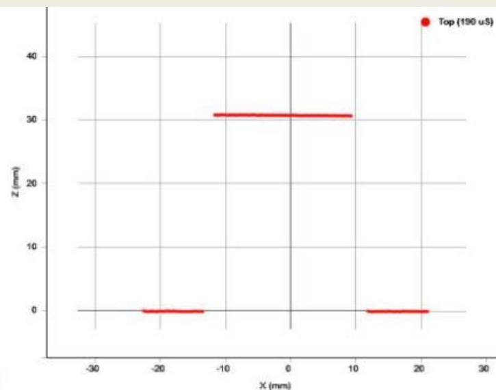
Výsledný laserový profil
